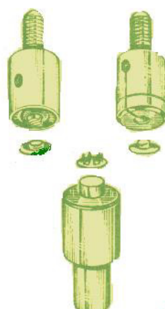
MATRIZ DE PRESSÃO Nº 35 / 38 Nº 35E / 38E
