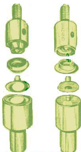
MATRIZ DE PRESSÃO Nº 80 - 100
